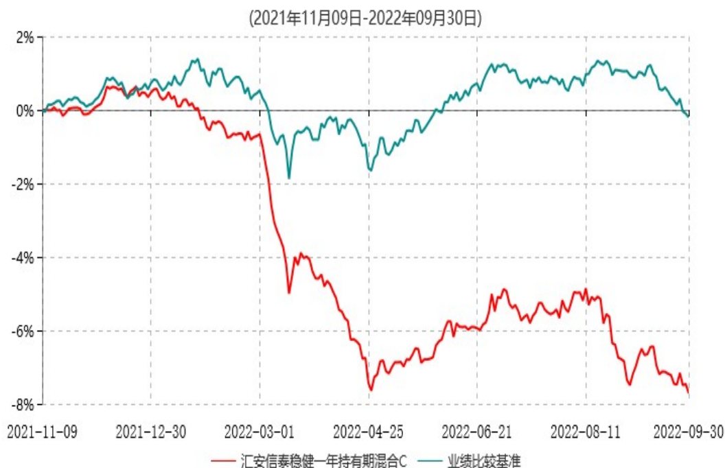
汇安信泰稳健一年持有期混合C累计净值增长率与业绩比较基准收益率历史走势对比图
